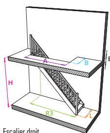
Escalier droit
